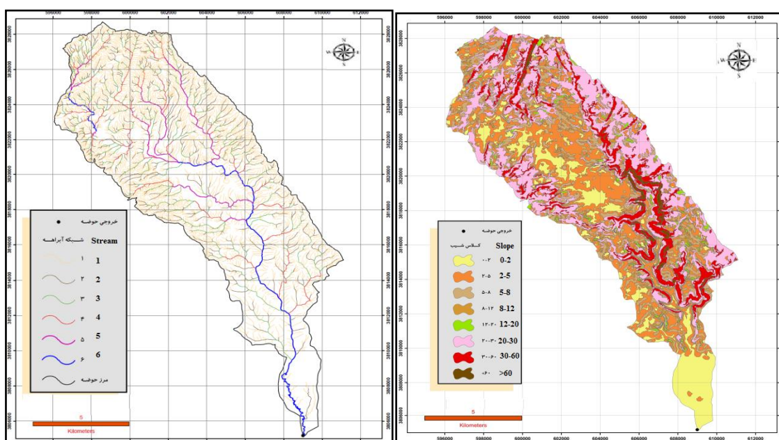
شکل ۷- نقشه شیب
