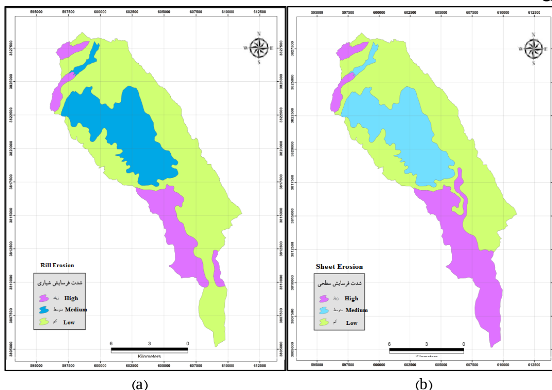
شکل ۸- نقشه شدت فرسایش حوضه زیمکان با مقایسه دوروش EPM (a) و MPSIAC (b)
