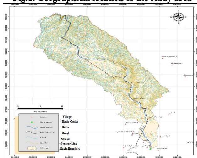
شکل ۲- نقشه پایه منطقه مود مطالعه
