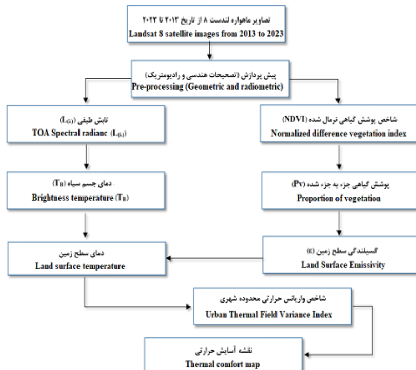
شکل ۲- مراحل محاسبه دمای سطح زمین و شاخص واریانس حرارتی محدوده شهری برای آسایش حرارتی
