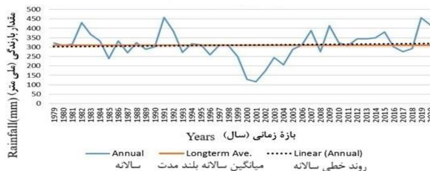
شکل ۴- میانگین سالانه درازمدت بارندگی در حوضه آبریز کابل از ۱۹۷۹-۲۰۲۰
