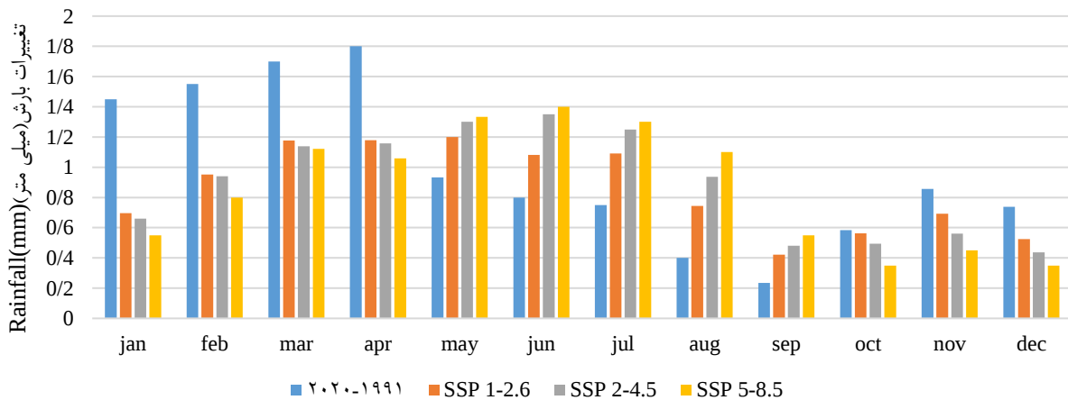
شکل ۱۰- میانگین بارش ماهانه پیش‌بینی شده در مقایسه با دوره پایه ایستگاه عمرض با استفاده از سناریوهای مدل
