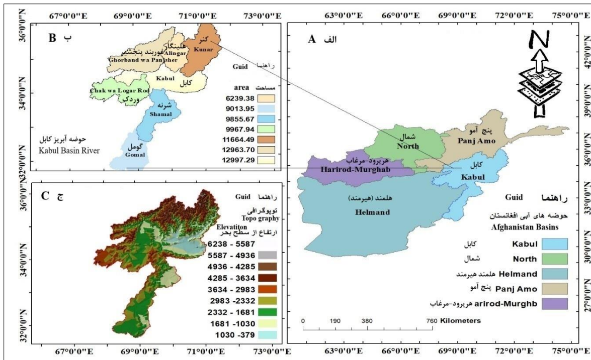
شکل ۱- الف) حوضه‌های آبی افغانستان، ب) منطقه مورد مطالعه ج) توپوگرافی
