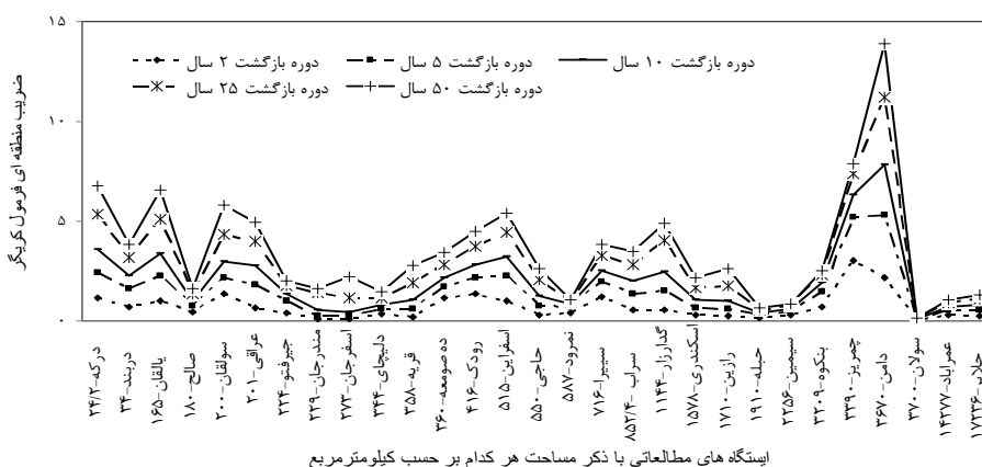
شکل ۲ ضریب منطقه‌ای فرمول کریگر با دوره بازگشت‌های ۲ و ۵۰ ساله در ایستگاه‌های مطالعاتی به ترتیب مساحت (کیلومتر مربع)
