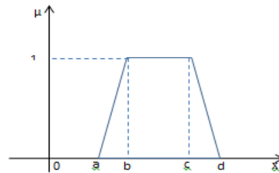
شکل ۶- نحوه نمایش اعداد ذوزنقه‌ای فازی
