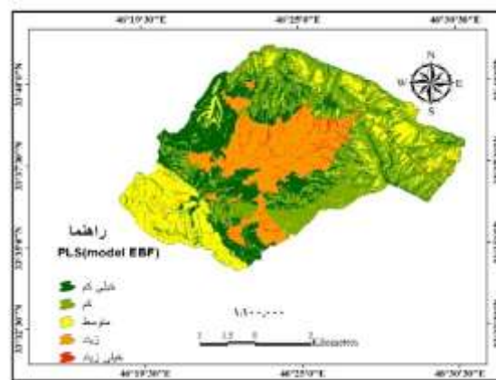
تابع احتمال
