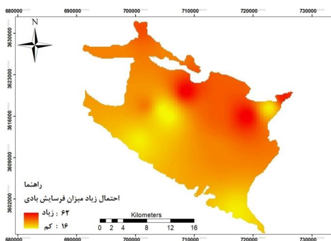
شکل ۶- نشان دهنده نقشه احتمالات زیاد میزان فرسایش بادی در منطقه مورد مطالعه
