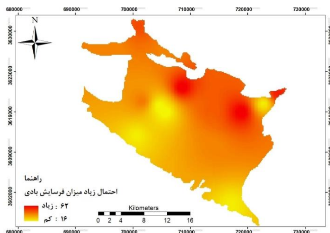
شکل ۳ - کلاس بندی فرسایش بادی در منطقه مورد مطالعه با استفاده از معیار فرسایش بادی مدل IMDPA
