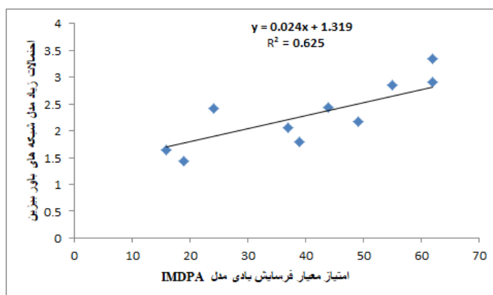
شکل ۷- نشان‌دهنده همبستگی بین امتیاز معیار فرسایش بادی در مدل IMDPA و احتمالات زیاد پیش‌بینی شده برای مدل شبکه‌های باور بیزین.
