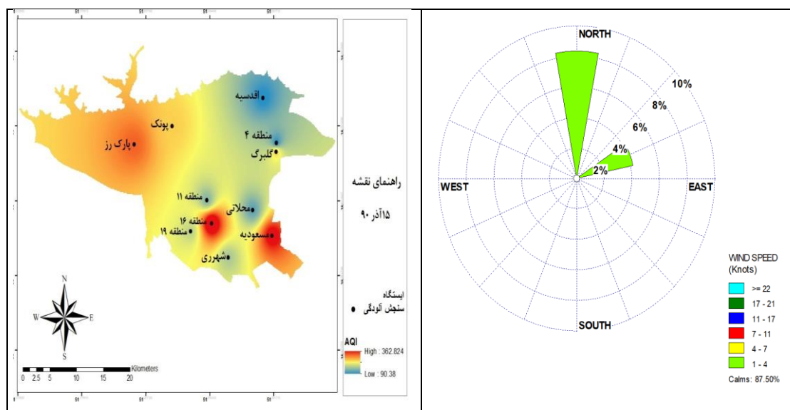
شکل ۲- بررسی وضعیت ایستگاه‌های آلوده سنجی شهر تهران و گلباد ایستگاه چیتگر در تاریخ ۶ دسامبر
