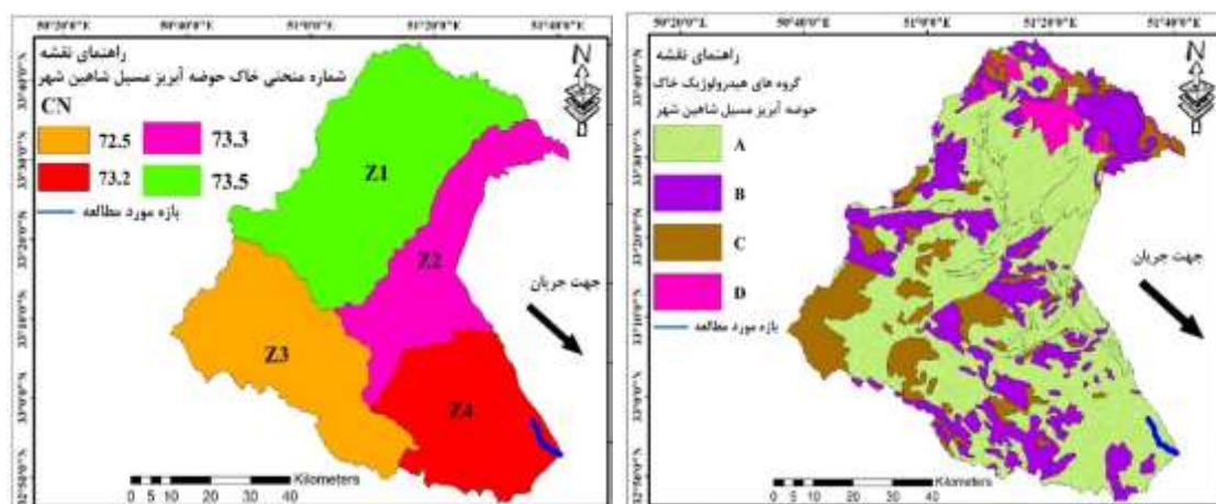
شکل ۶- گروه‌های هیدرولوژیک خاک حوضه
