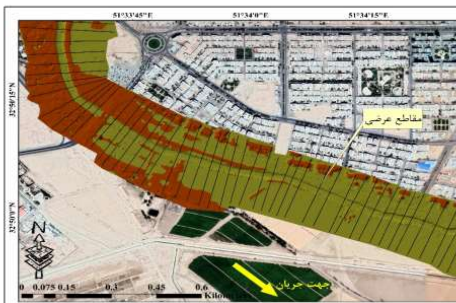
شکل ۲- بخشی از TIN مسیل شاهین شهر و مقاطع عرضی در محیط GIS
