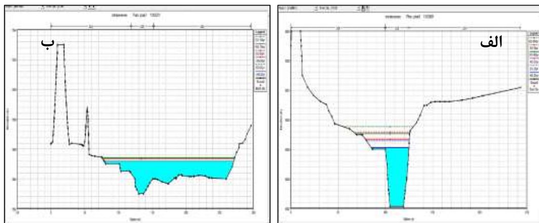
شکل ۱۱ الف و ب- مقطع عرضی مسیل شاهین شهر در دوره بازگشت ۲۵، ۵۰ و ۱۰۰سال و پهنه سیلاب در دوره بازگشت ۲۵، ۵۰، ۱۰۰-
