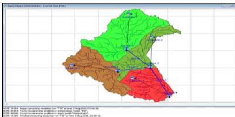
شکل ۸- شماتیک تعیین حداکثر دبی عبوری مسیل شاهین شهر بر اساس حداکثر دبی خروجی هر یک از زیرحوضه‌ها
