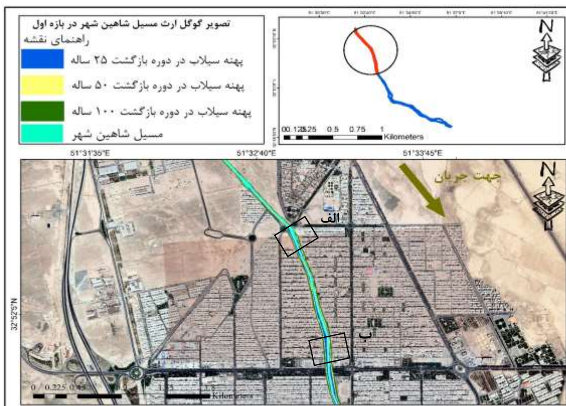
شکل ۹- نقشه پهنه بندی سیلاب مسیل شاهین شهر در دوره بازگشت ۲۵ و ۵۰ و ۱۰۰ ساله
