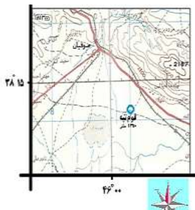
شکل ۲- موقعیت قوم تپه صوفیان در نقشه‌های توپوگرافی و زمین شناسی
