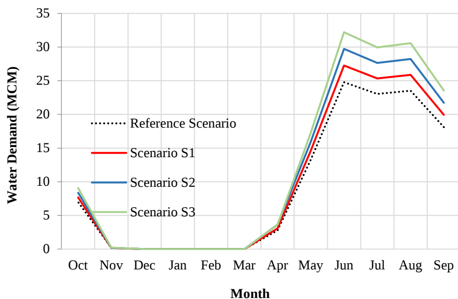
شکل ۸- میزان تقاضای کشاورزی در سناریوهای مرجع و افزایش سطح زیر کشت (MCM) Fig.8. Agricultural water demand in the reference and cultivated area expansion scenarios (MCM)
