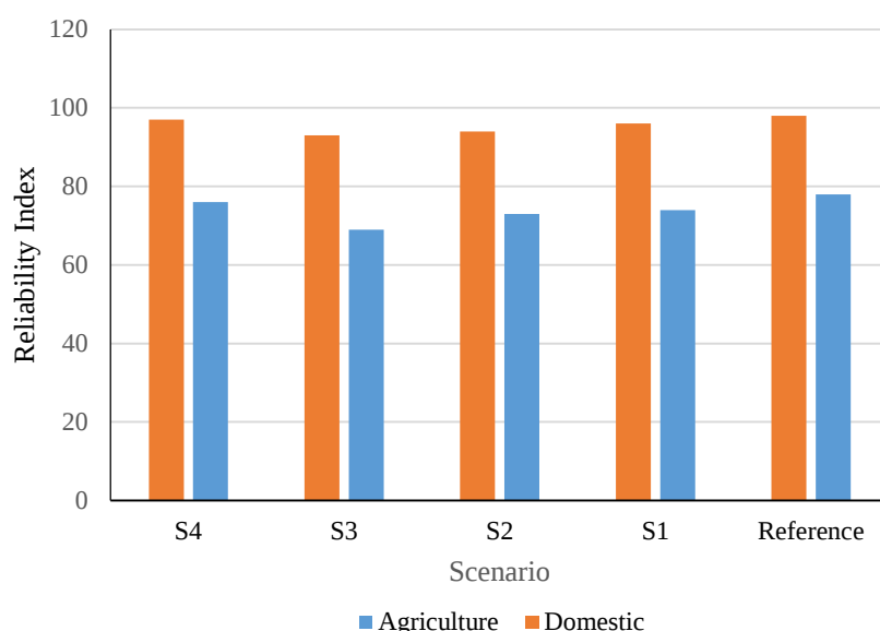
شکل ۱۲- شاخص اطمینان پذیری بر حسب درصد در سایت های کشاورزی و شهری
