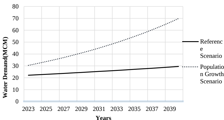
شکل ۱۰- میزان تقاضای شهر مهاباد در سناریوهای مرجع و افزایش نرخ رشد جمعیت (MCM) Fig.10. Water demand of Mahabad City in the reference and population growth rate increase scenarios (MCM)
