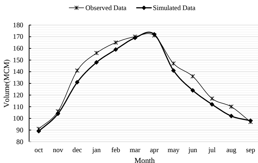
شکل ۵- مقایسه مقادیر مشاهده‌ای و شبیه‌سازی حجم مخزن سد مهاباد بر حسب میلیون مترمکعب Fig. 5. Comparison between observed and simulated reservoir of Mahabad Dam's volume (in million cubic meters)
