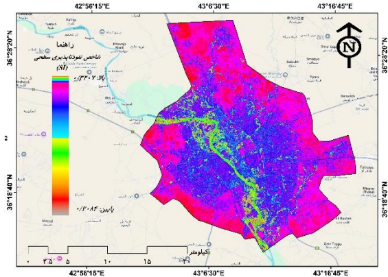
شاخص نفوذناپذیری سطحی
