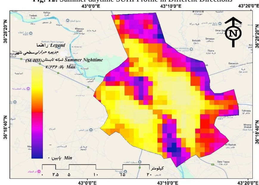
شکل ۱۳- شاخص SUHI شبانه تابستان ۱۴ ژوئیه
