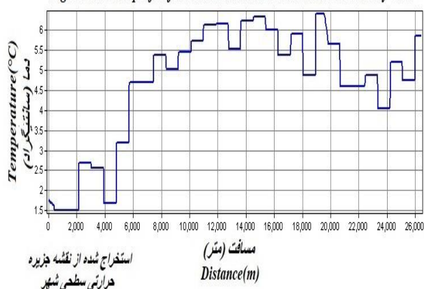
پروفیل جزیره حرارتی سطحی شهر در طول شب از شمال به جنوب شهر موصل ۱۴ ژوئیه ۲۰۲۴ Nighttime SUHI profile from north to south across Mosul on 14 July 2024
