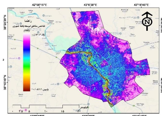
شاخص بر مبنای مناطق ساخته شده (IBI)
