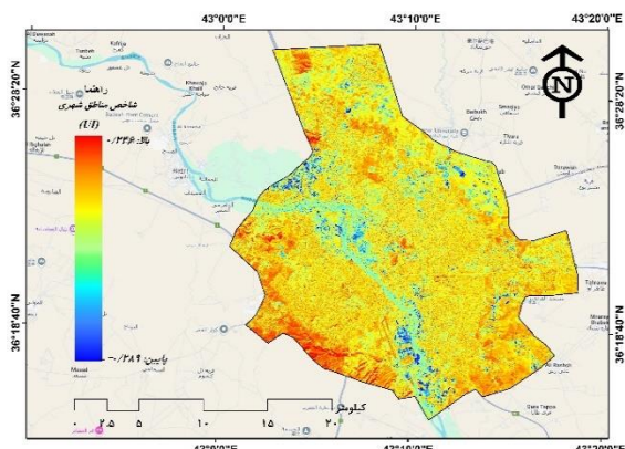
شاخص مناطق شهری (UI)
