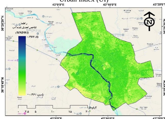
شاخص تعدیل شده آب (MNDWI)
