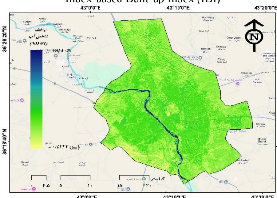
شاخص تفاوت نرمال شده آب (NDWI)
