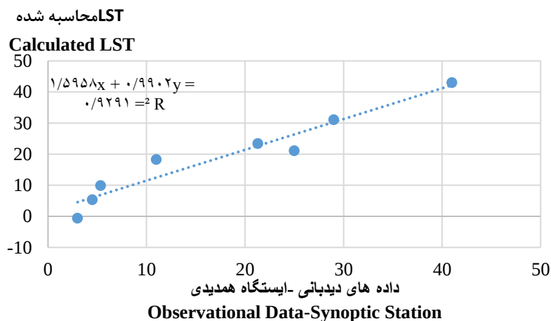
شکل ۸- همبستگی بین داده های ایستگاه همدیدی و دمای سطح زمین
