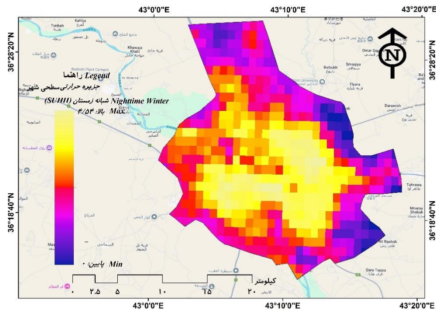
شکل ۱۷- شاخص SUHI شبانه زمستان ۲۵ ژانویه
