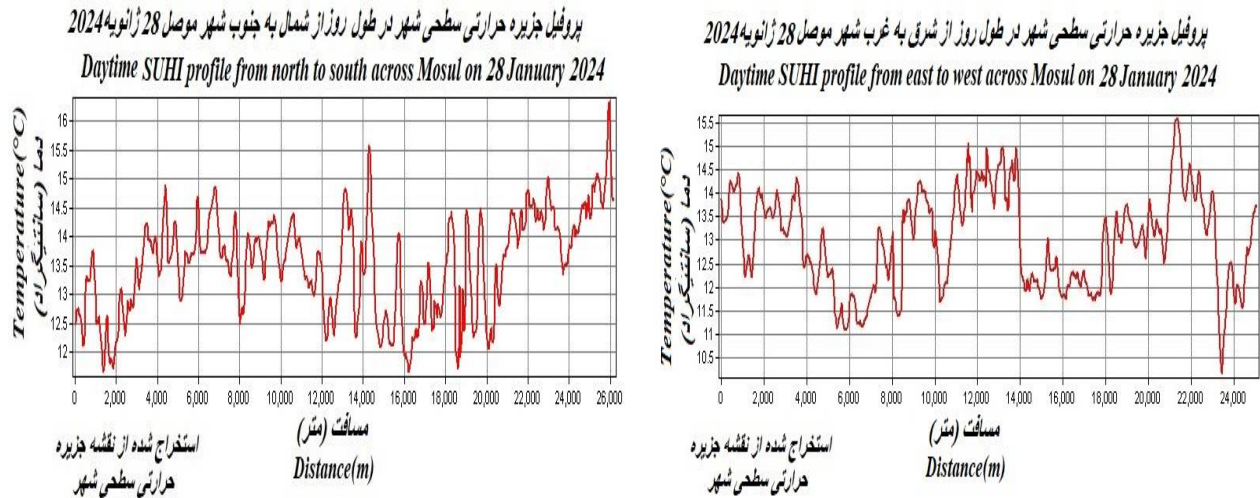
ب-جزیره حرارتی روزانه شمال به جنوب روزانه ۲۸ ژانویه b. Daily heat island from north to south – January 28 الف-جزیره حرارتی روزانه از شرق به غرب ۲۸ ژانویه a. Daily heat island from east to west – January 28
