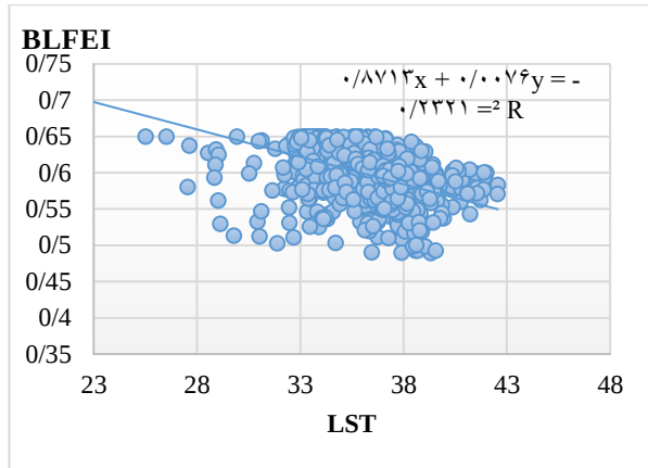
الف. رابطه همبستگی بین BLFEI و LST a. Correlation between BLFEI and LST
