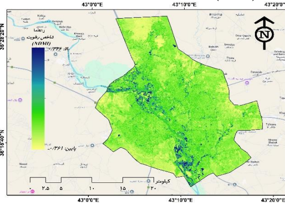
شاخص رطوبت (NDMI)
