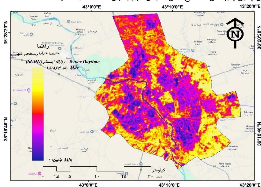
شکل ۱۵- شاخص SUHI روزانه زمستان ۲۸ ژانویه
