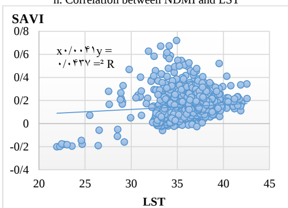
د. رابطه همبستگی بین LST و SAVI j. Correlation between SAVI and LST
