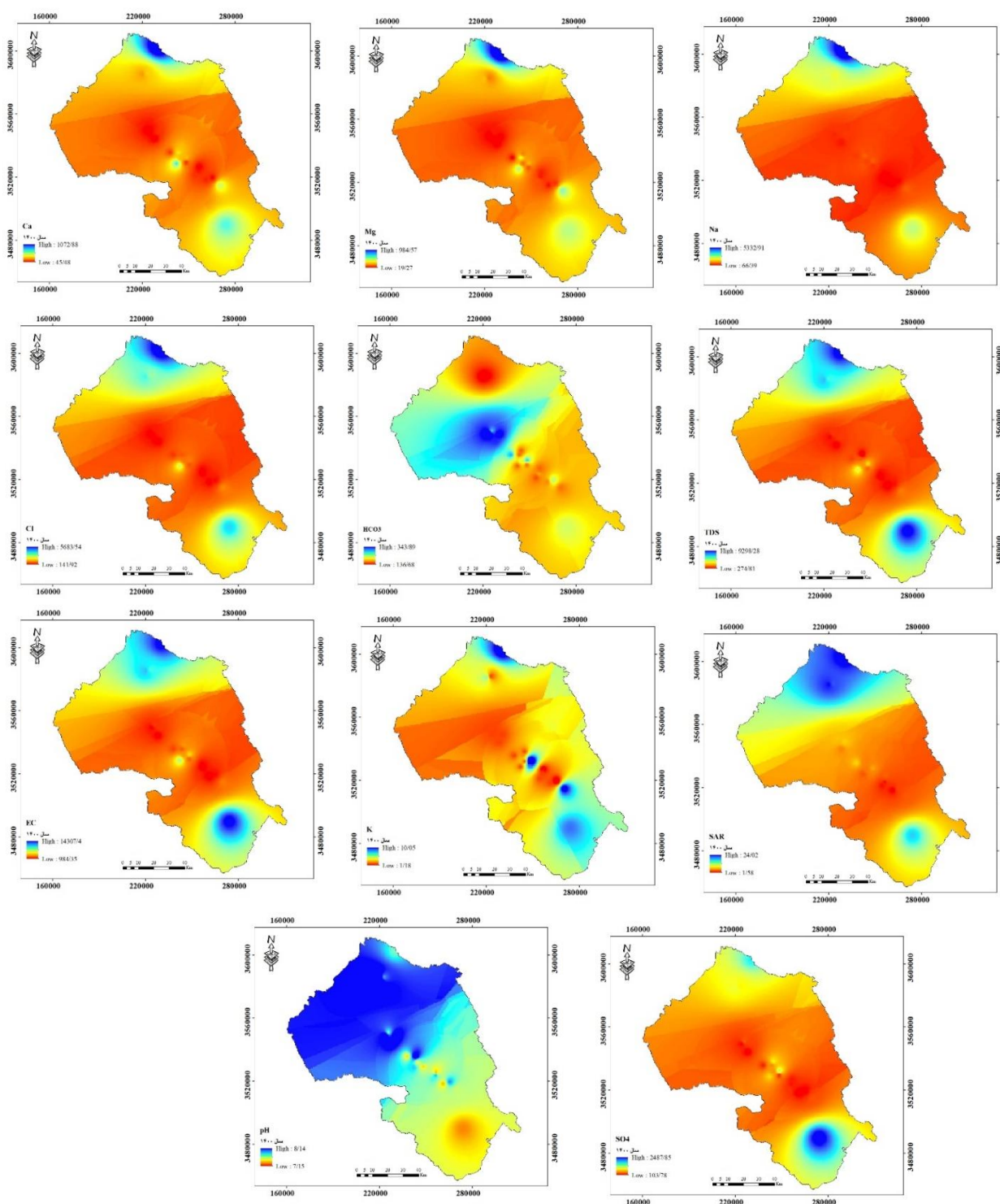
شکل ۳- پهنه‌بندی غلظت کاتیون‌ها، آنیون‌ها، شوری، مواد جامد محلول، pH و نسبت جذب سدیم در دشت یزد - اردکان در سال ۱۴۰۰ Fig. 3. Zoning of the concentration of cations, anions, salinity, dissolved solids, pH and SAR in the Yazd-Ardakan plain in 2021
