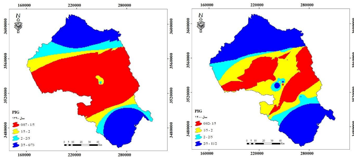
شکل ۶- پهنه‌بندی شاخص PIG در سال ۱۳۹۰ و ۱۴۰۰ در دشت یزد اردکان
