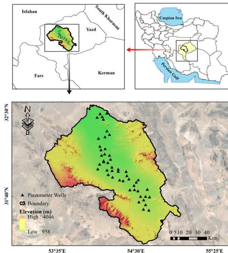
شکل ۱- موقعیت دشت یزد - اردکان و چاه‌های پیزومتری
