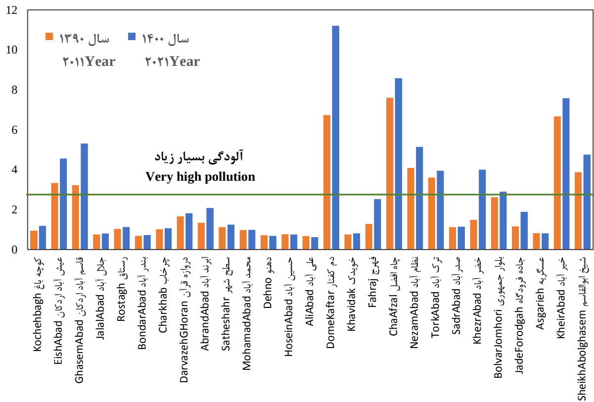
شکل ۵- مقادیر شاخص PIG در دو سال ۱۳۹۰ و ۱۴۰۰ در ۲۷ چاه مورد بررسی
