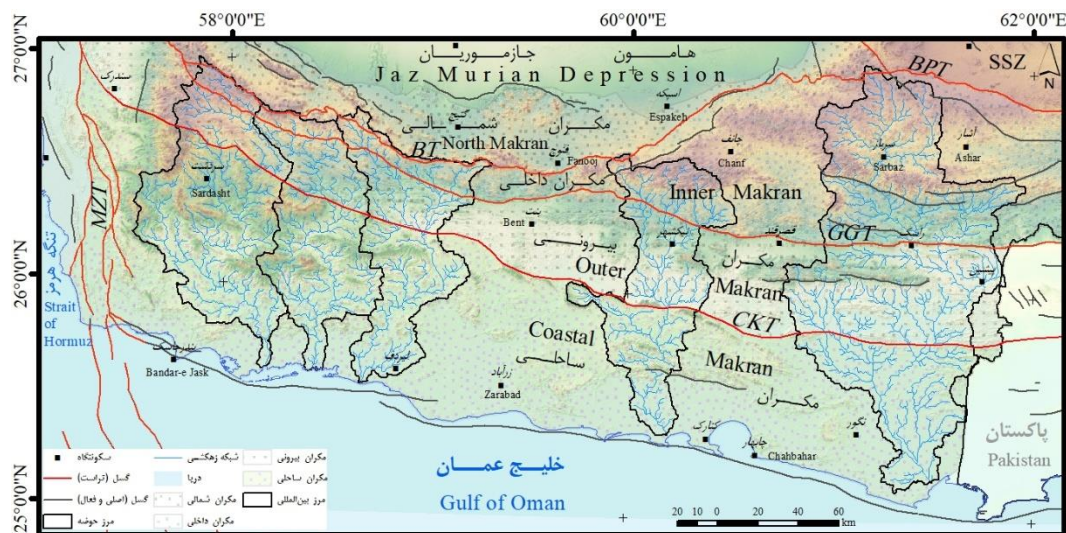
شکل ۲- موقعیت حوضه های منطقه مورد مطالعه در منشور برآزایشی مکران (به ترتیب از راست به چپ: باهوكلات، كهپر، سدیح، گابریك و جگین). اطلاعات موجود بر روی این شكل، با شكل ۱ ب یکسان است؛ برای اطلاعات بیشتر به آن مراجعه كنید.
