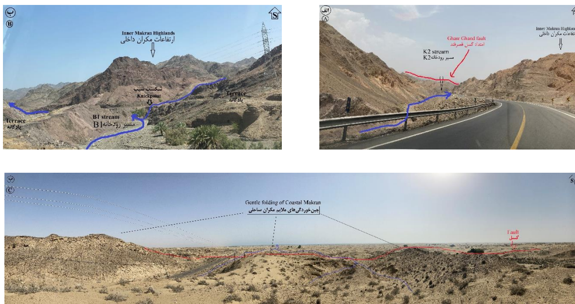
شکل ۷- تصاویر میدانی از چشم‌انداز ژئومورفیک حوضه‌های مورد مطالعه. الف) آبراه شماره دو حوضه کهیر، ب) آبراه شماره یک حوضه باهوکلالت، پ) پایاب حوضه سدیچ (آبراه شماره چهار).
