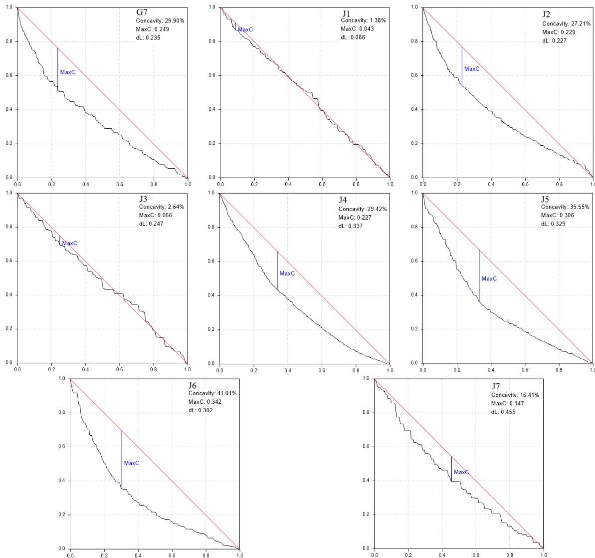
شکل ۱۰- نیمرخ‌های طولی نرمال‌شده برای آبراهه‌های فرعی در حوضه‌های پنج‌گانه (B: باهوكلات، K: كهير، S: سديچ، G: گابريك، J:
