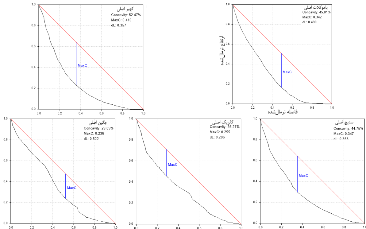
شکل ۸- نیمرخ‌های طولی نرمال‌شده برای آبراهه‌های اصلی حوضه‌های پنج‌گانه. برای آگاهی از موقعیت مکانی، به شکل مراجعه کنید.
