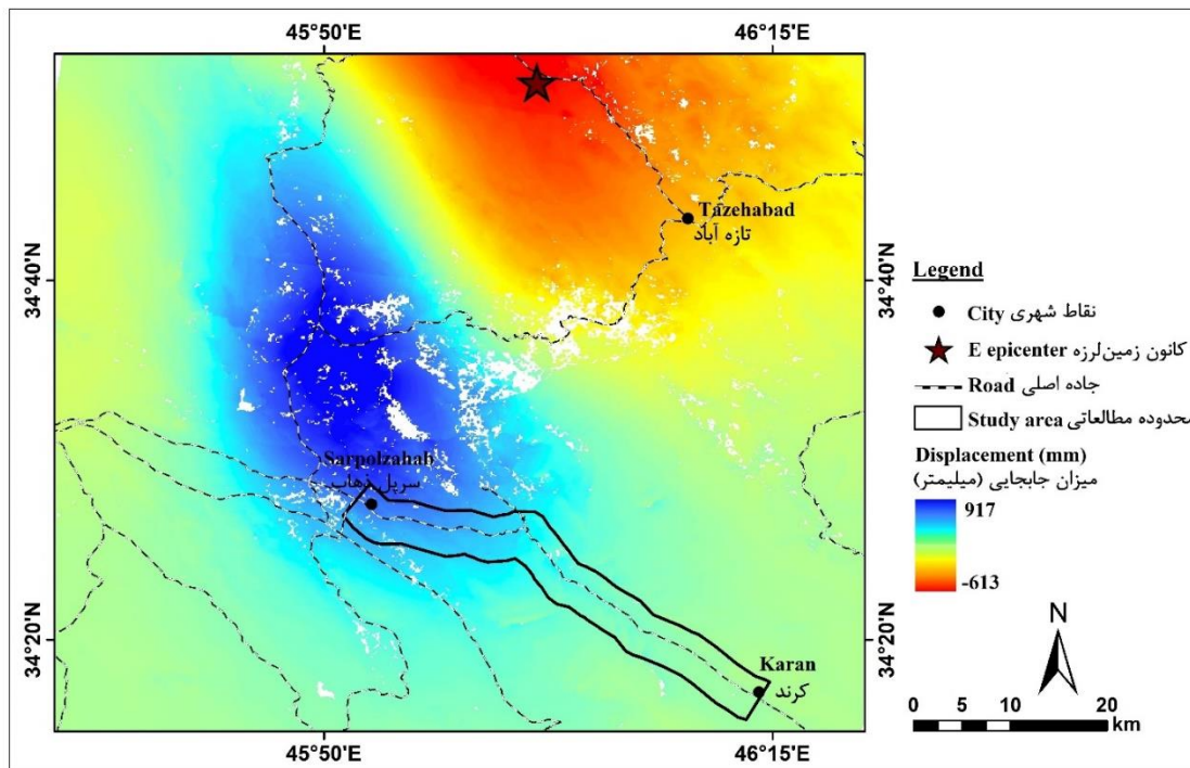
شکل ۶- نقشه میزان جابه‌جایی عمودی منطقه
