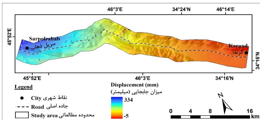
شکل ۷- نقشه میزان جابه‌جایی عمودی محدوده مطالعاتی تحت تأثیر زمین‌لرزه از گله
