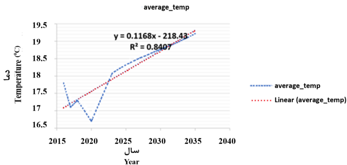
شکل ۹- پیش‌بینی دما تا سال ۲۰۳۵ با استفاده از مدل LSTM
