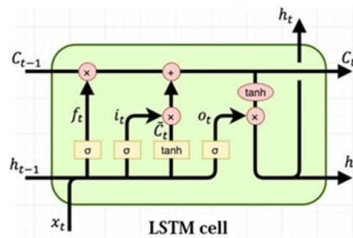
شکل ۷- ساختار داخلی سلول LSTM و نحوه‌ی جریان اطلاعات بین اجزای آن
