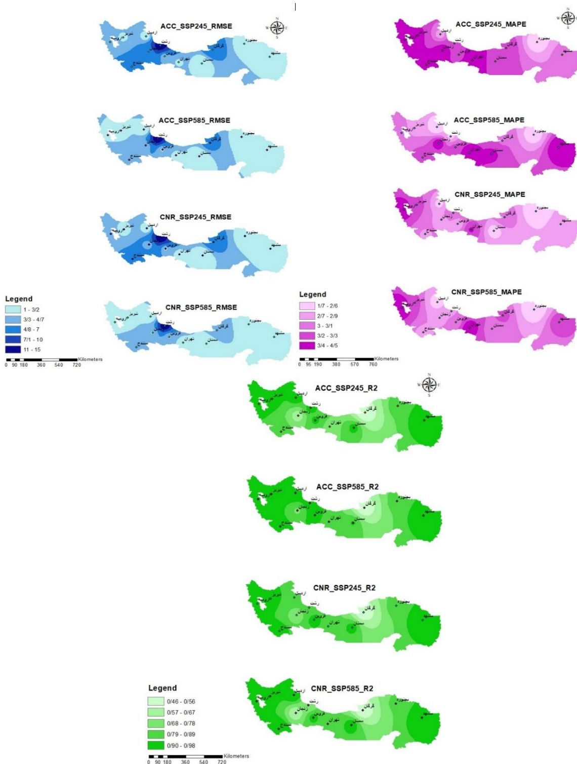
شکل ۷- نقشه‌های پراکندگی دقت سناریوهای دو مدل در پیش‌نمایی بارش ۲۰ سال آبی ایستگاه‌ها (۲۰۴۱-۲۶۰) Fig.7. Accuracy maps of two models in precipitation forecasting, based on three indices: R2, MAPE, RMSE (2041-260)
