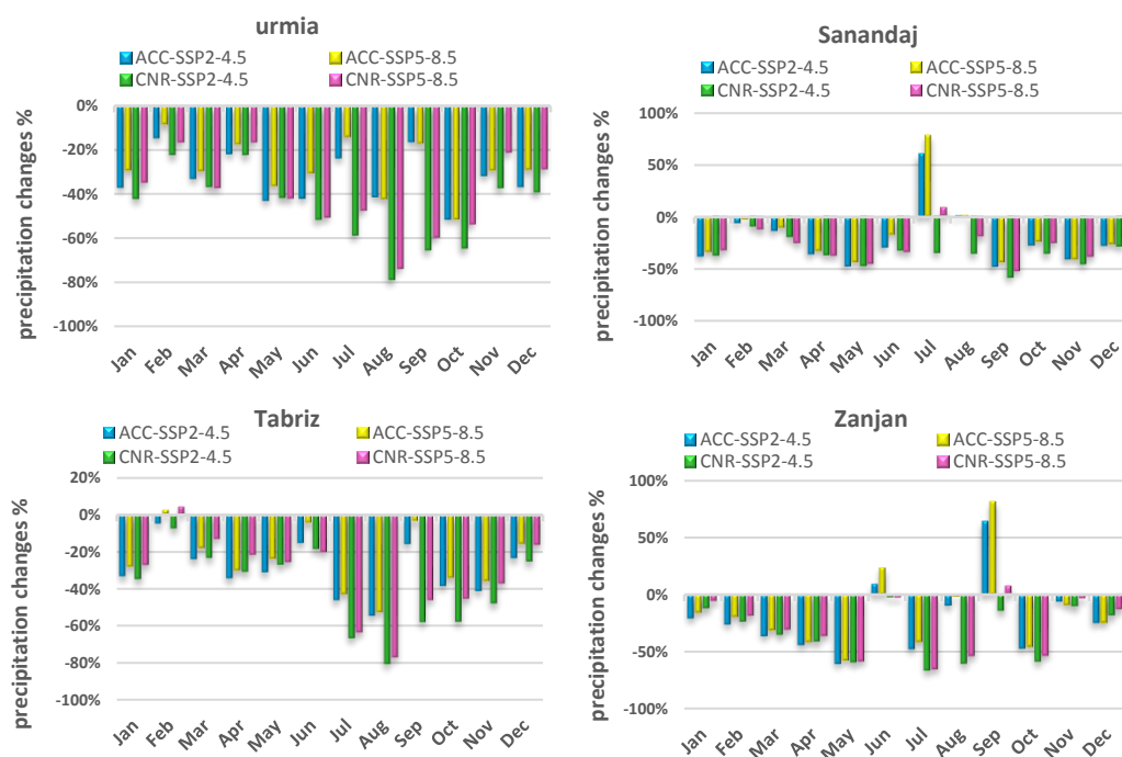
شکل ۶- نمودارهای درصد تغییرات بارش پیش‌بینی‌شده بر اساس سناریوهای دو مدل ACCESS و CNRM (۲۰۴۱-۲۰۶۰)
