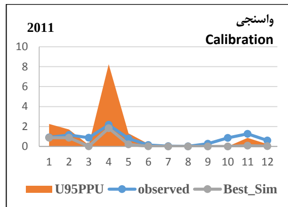
شکل ۹- منحنی رابطه رواناب مشاهده‌ای و شبیه‌سازی شده منطقه در دوره واسنجی ۲۰۰۲-۲۰۰۹
