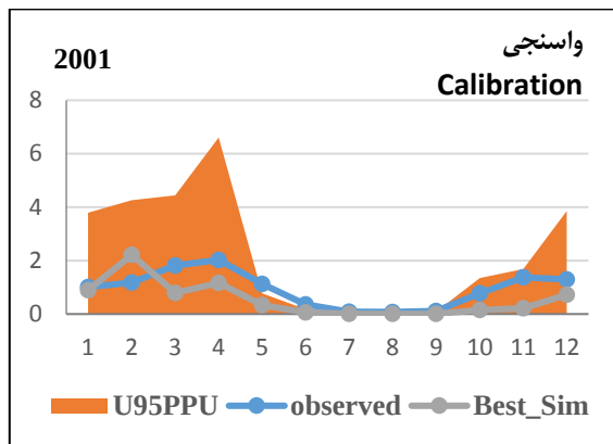
شکل ۸- منحنی رابطه رواناب مشاهده‌ای و شبیه‌سازی شده منطقه در دوره واسنجی ۱۹۸۵-۱۹۹۹
