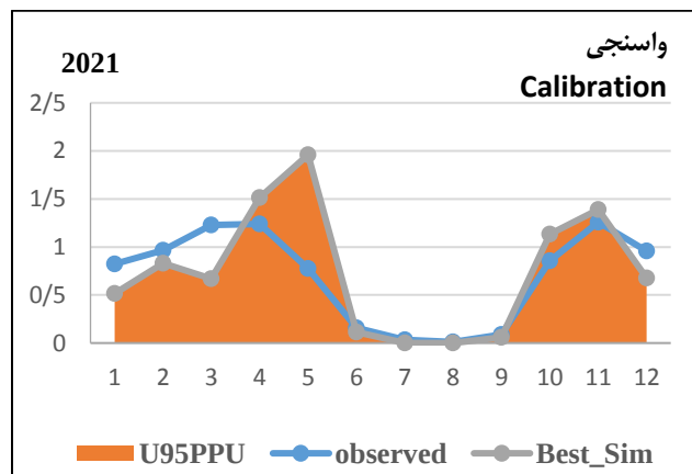
شکل ۱۰- منحنی رابطه رواناب مشاهده‌ای و شبیه‌سازی شده منطقه در دوره واسنجی ۲۰۱۲-۲۰۱۹
