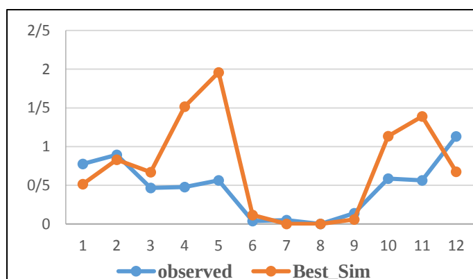
شکل ۱۳- منحنی رابطه رواناب مشاهده‌ای و شبیه‌سازی شده منطقه در دوره اعتبارسنجی ۲۰۲۰-۲۰۲۱
